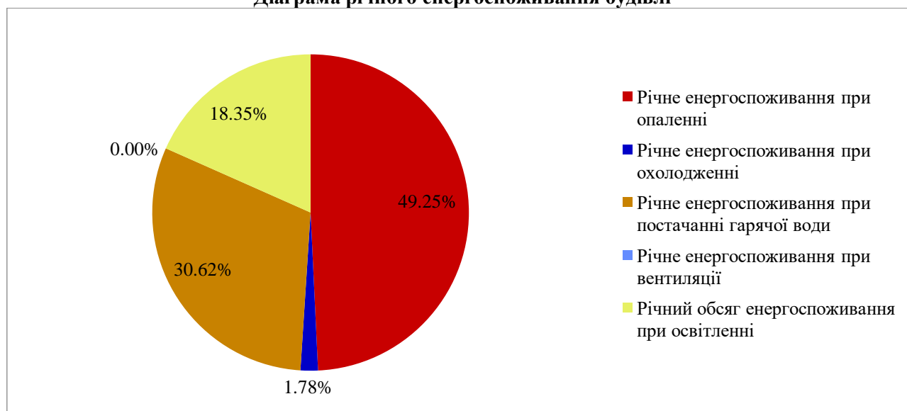
Діаграма річного енергоспоживання будівлі
